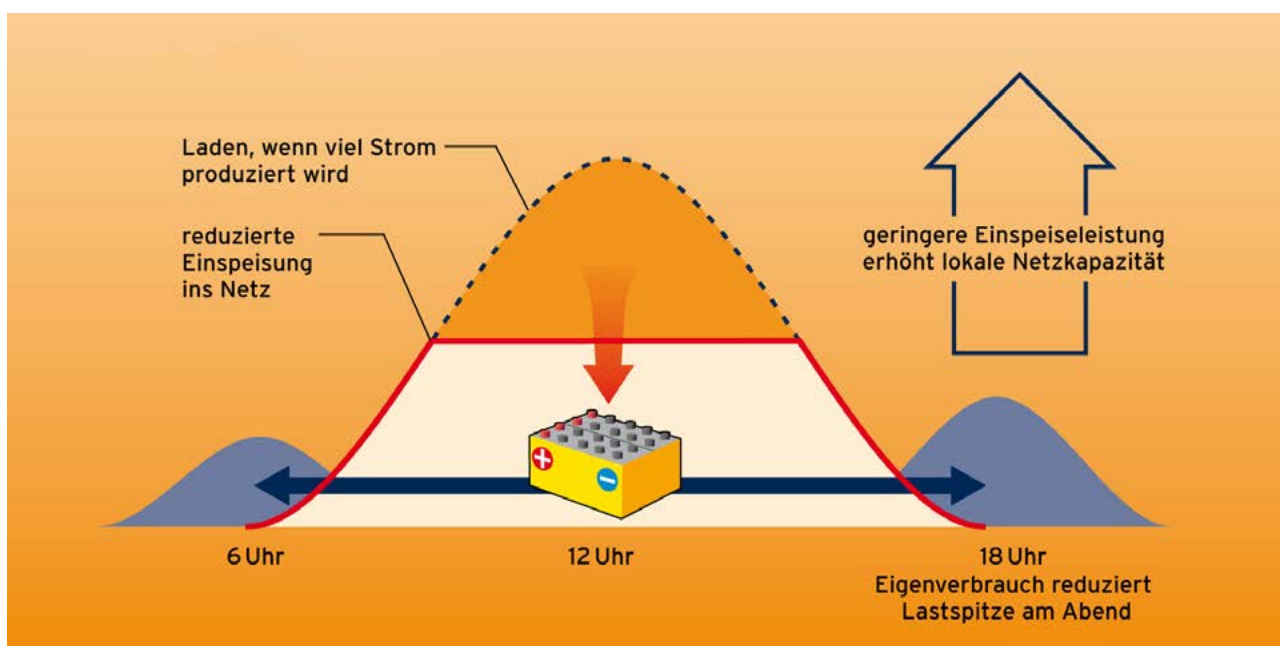
Wirkprinzip einer Batterie zur Erhöhung des Eigenstromverbrauchs (Quelle: Bundesverband Solarwirtschaft)
