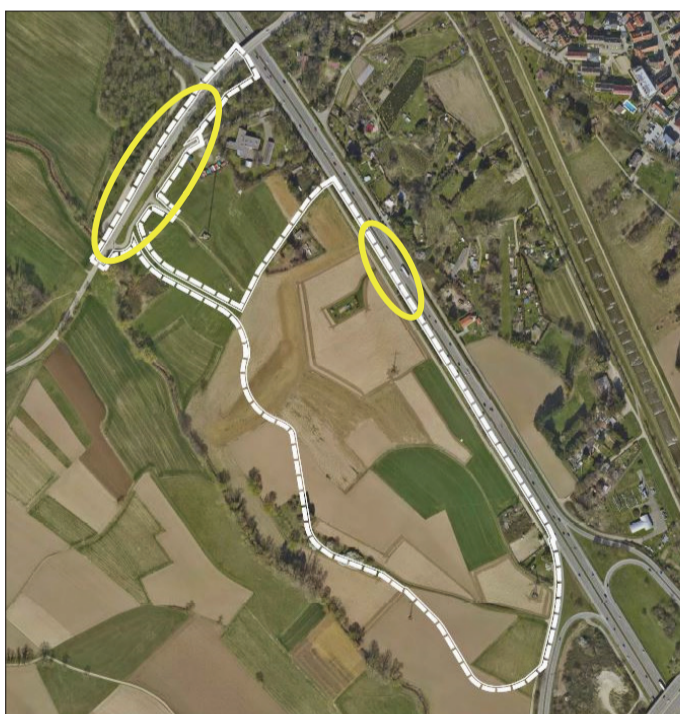
Rein und raus: Das Erdaushubzwischenlager im Dietenbach erhält getrennte Zu- und Abfahrten. (Plan: GuT)
